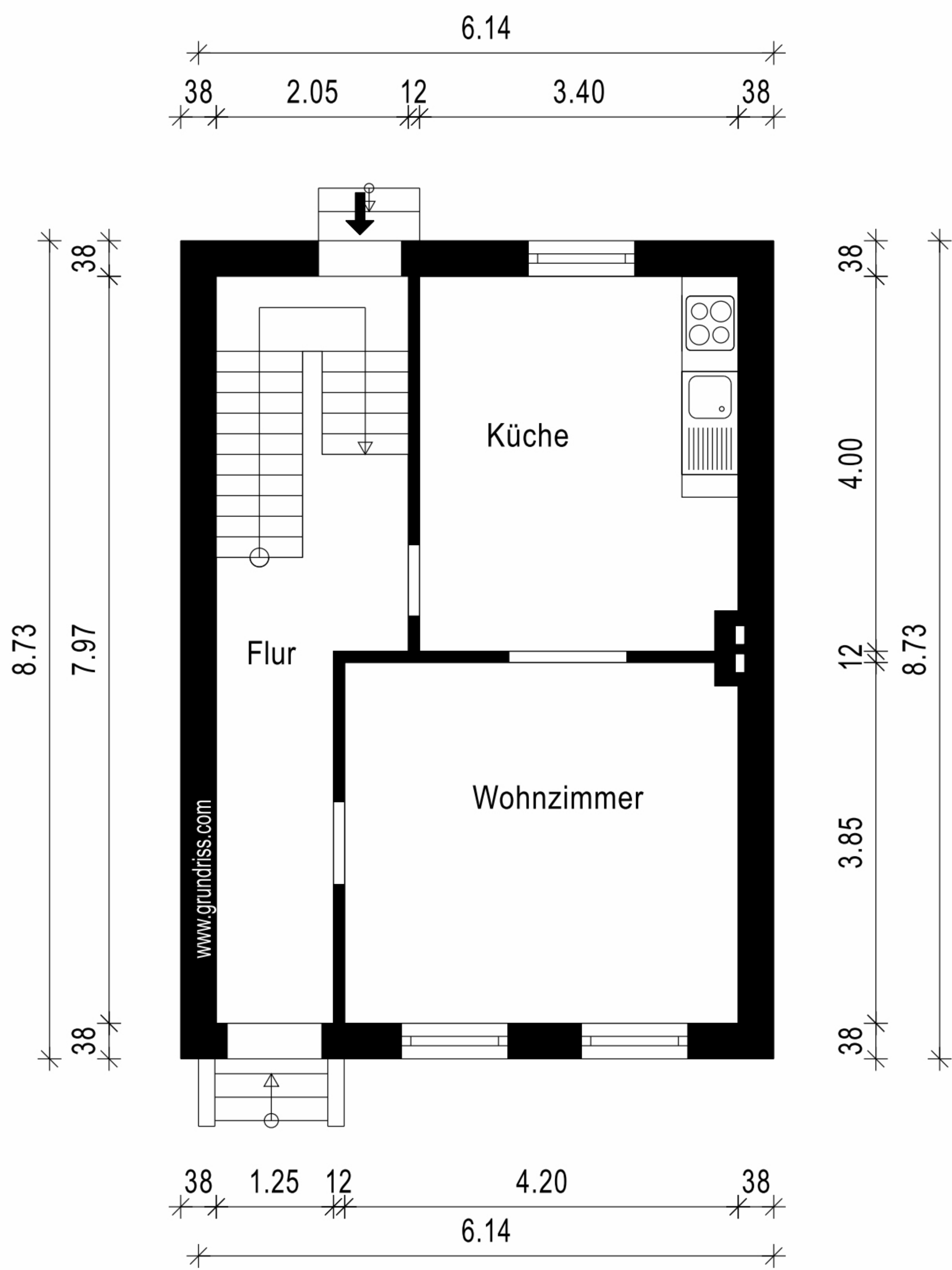
Erdgeschoss
