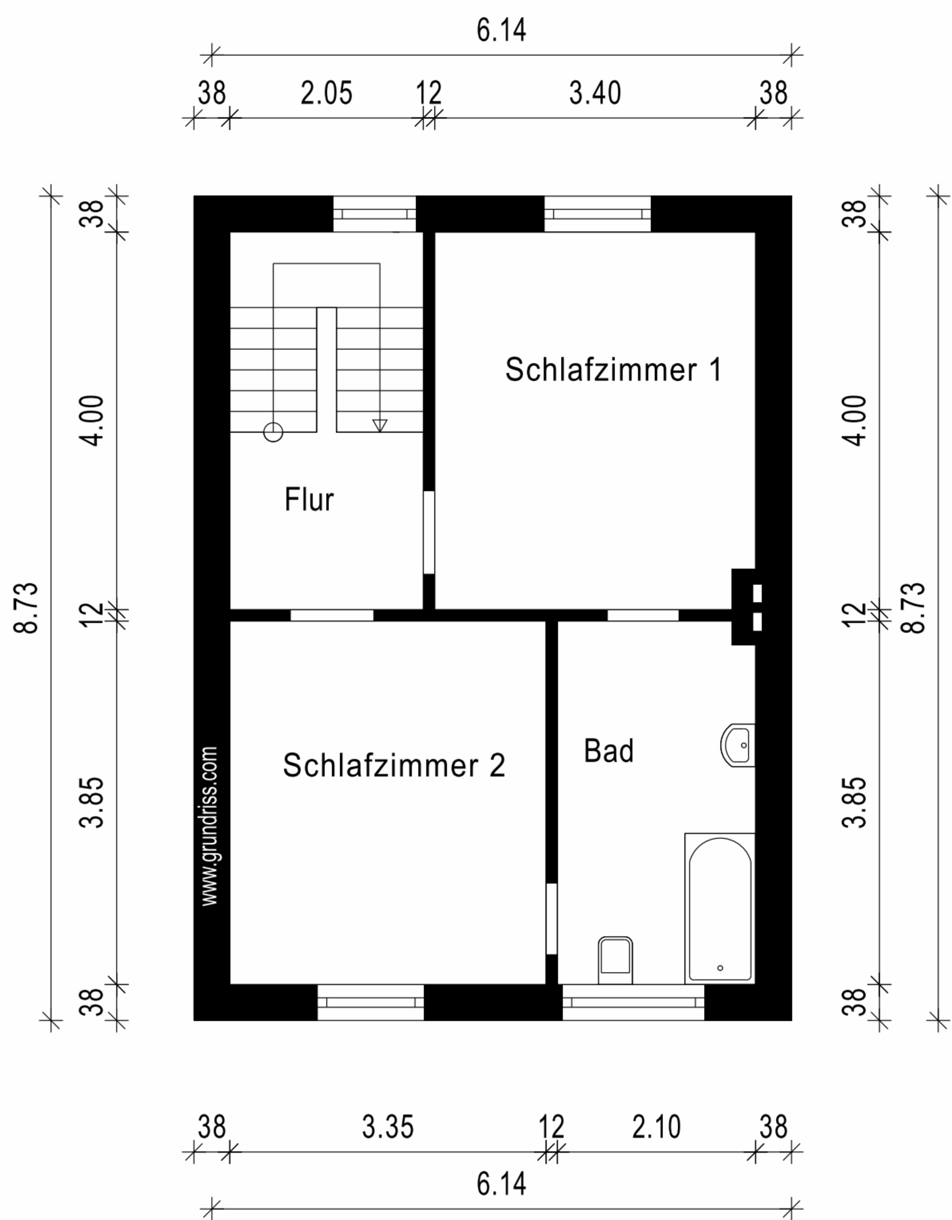
Obergeschoss
