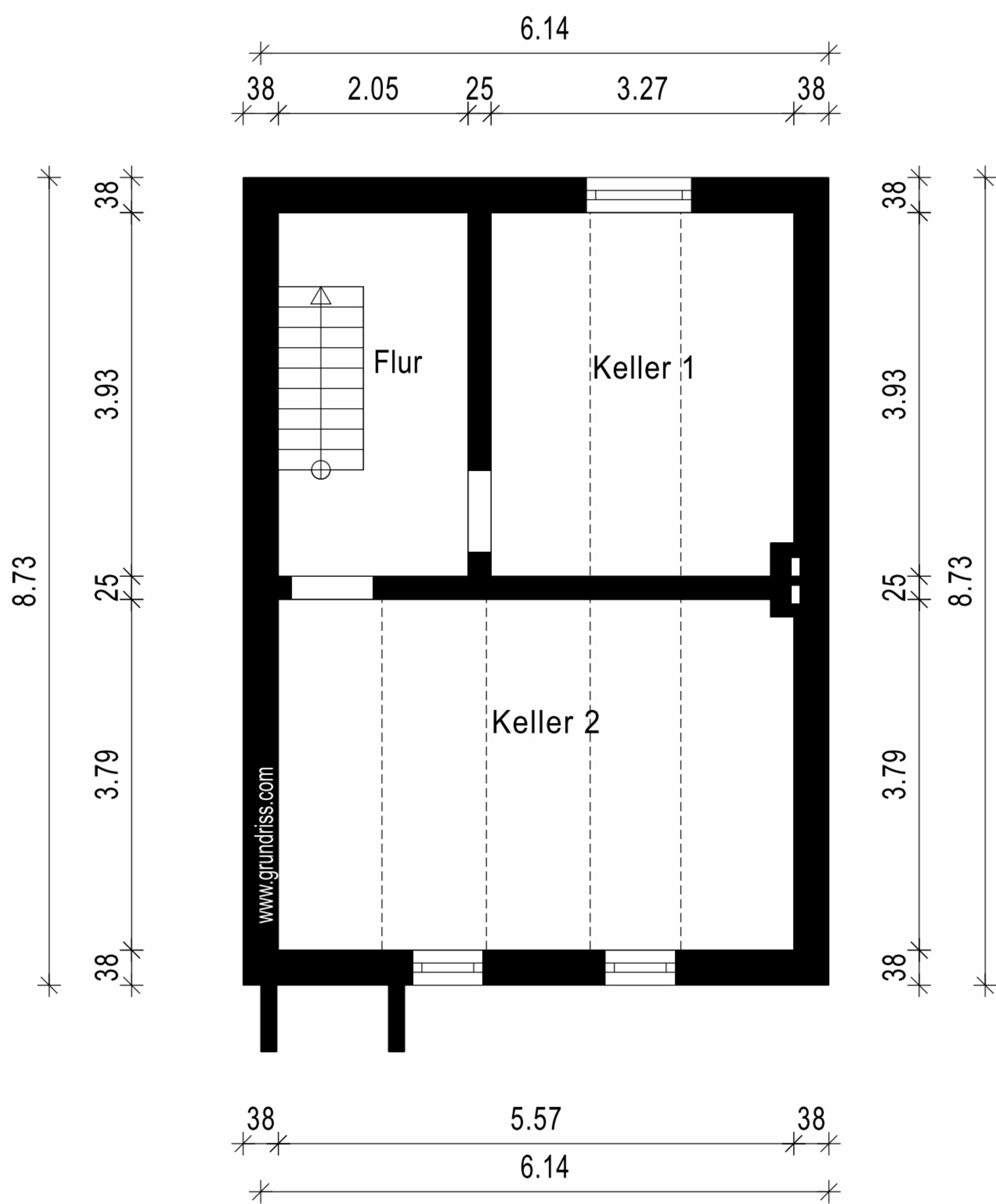
Kellergeschoss
